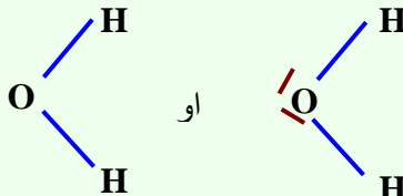
الصيغة المفصلة لـ \text{H}_2\text{O}
