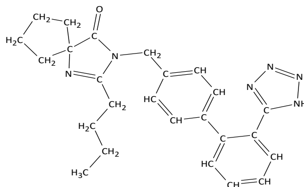
Irbesartan
